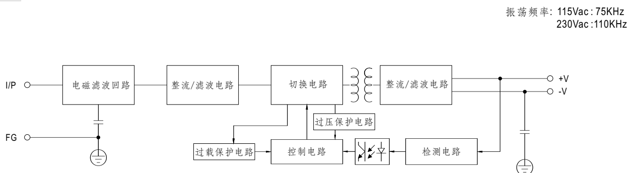
■ 方框图
