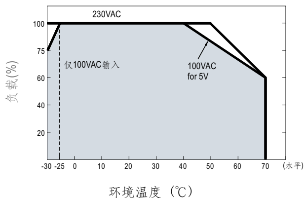
■ 减额曲线
