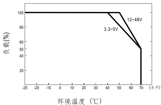
■ 减额曲线
