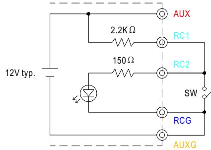
例3.2(C): 用内部12V辅助输出
