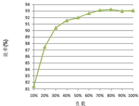
◎ 以上曲线是在230VAC下测得
