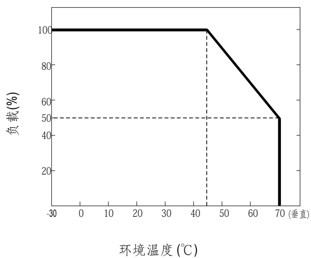
■ 减额曲线
