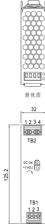
前视图
